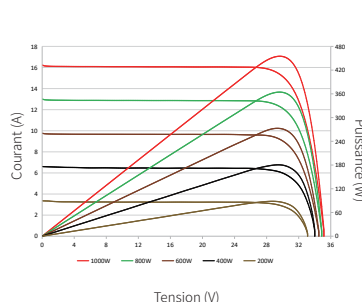
Courbes courant-tension et puissance-tension (445W)
